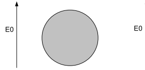
Figura 1.7: Esfera dielétrica em campo uniforme.
