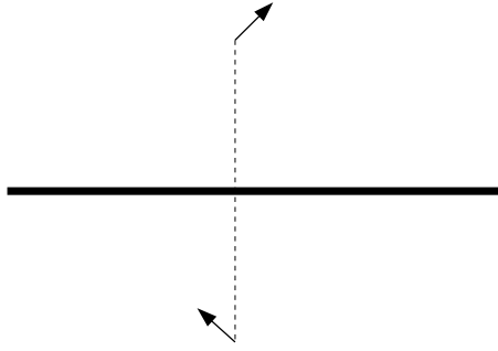
Figura 1.2: Dipolo imagem.
